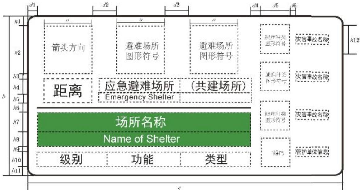
图 13 避难场所外指向标志(横版 2)尺寸参数
